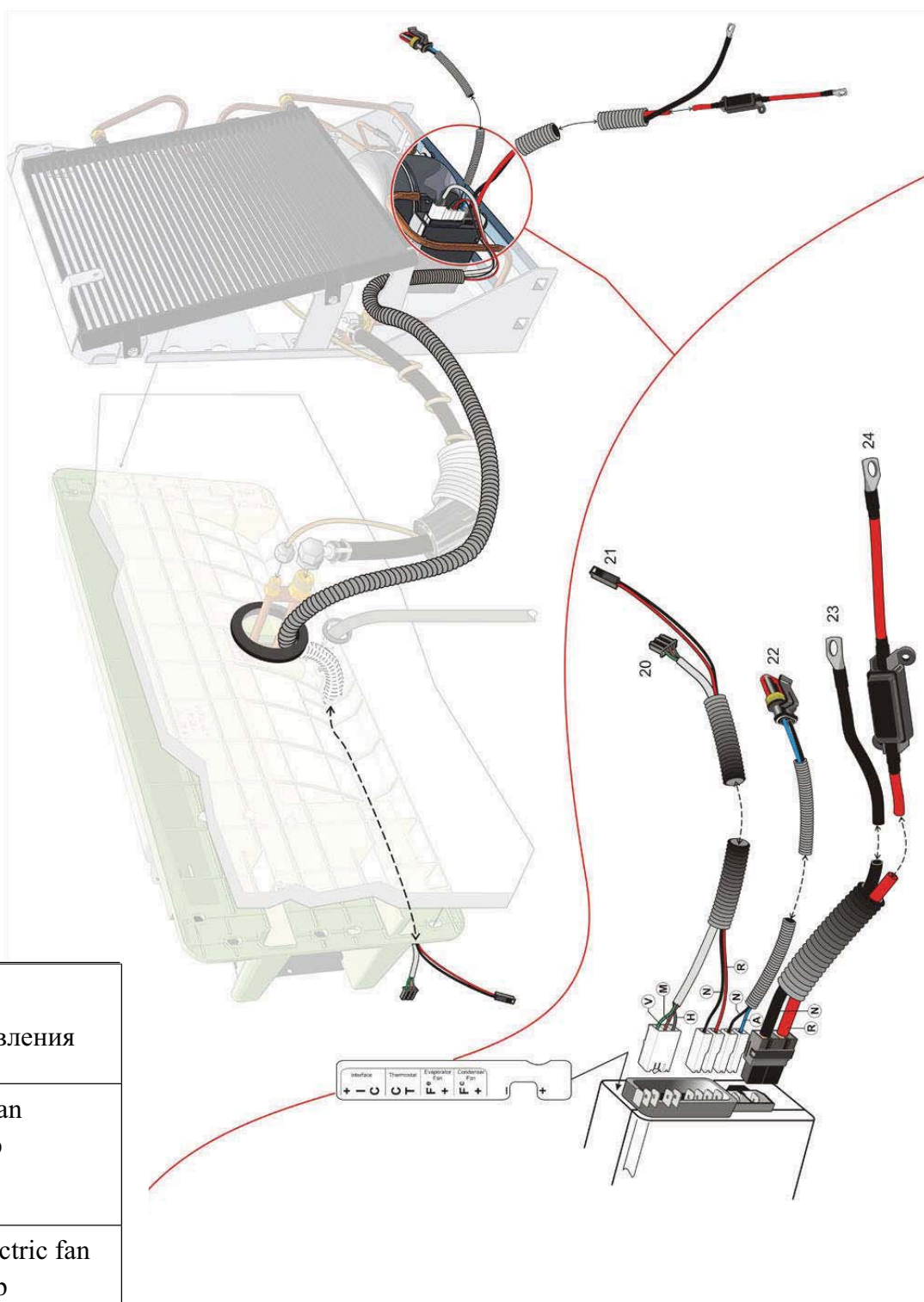
ELECTRICAL HARNESS WITH CONDENSER "BACK" ЭЛЕКТРО ПОДКЛЮЧЕНИЕ ВНЕШНЕГО ВЛОКА "BACK"
